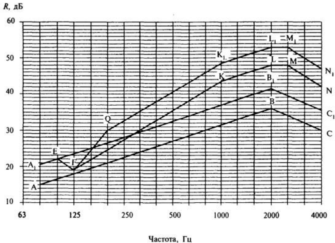
Рисунок 12 - Расчетная частотная характеристика к примеру 11
