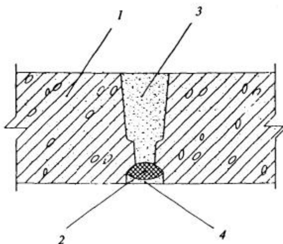
Рисунок 16 - Схема конструктивного решения узла примыкания двойной перегородки к перекрытию
