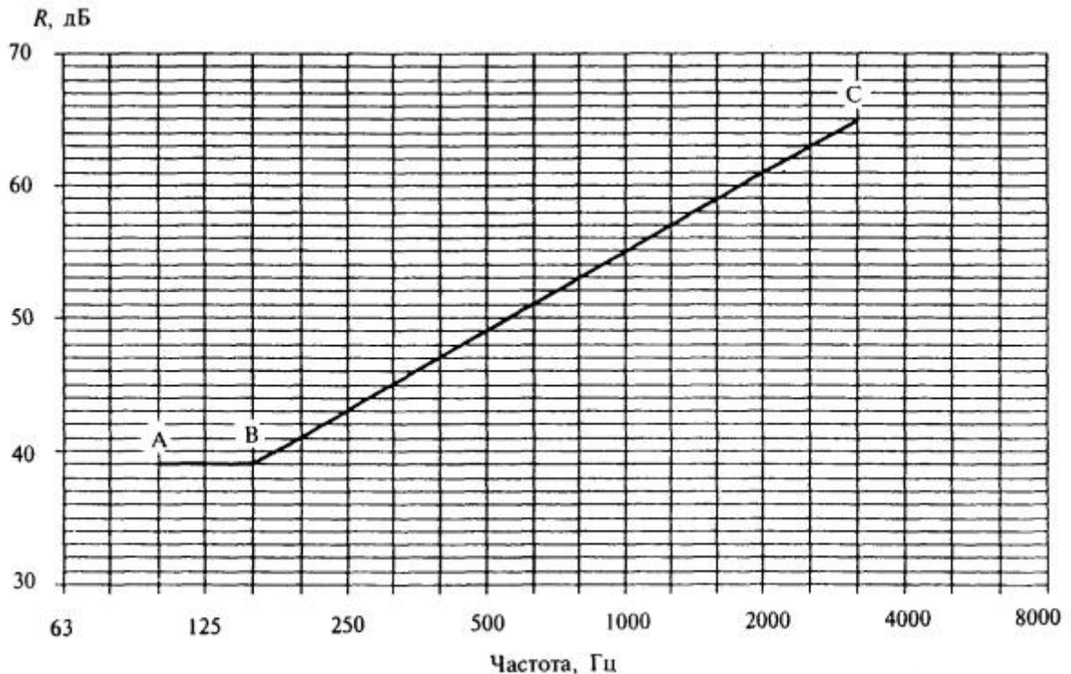
Рисунок 4 - Расчетная частотная характеристика к примеру 6
